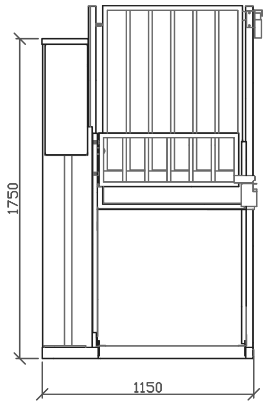
SIDOVY-kortsida
