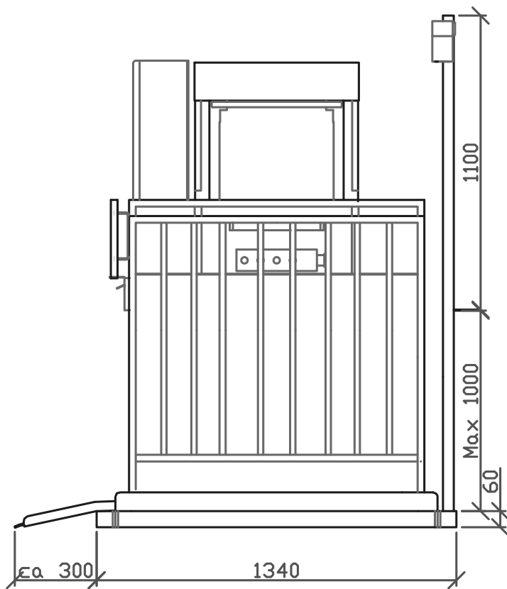
SIDOVY-långsida
